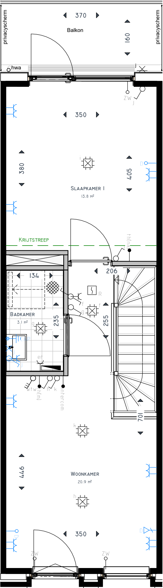
eerste verdieping
